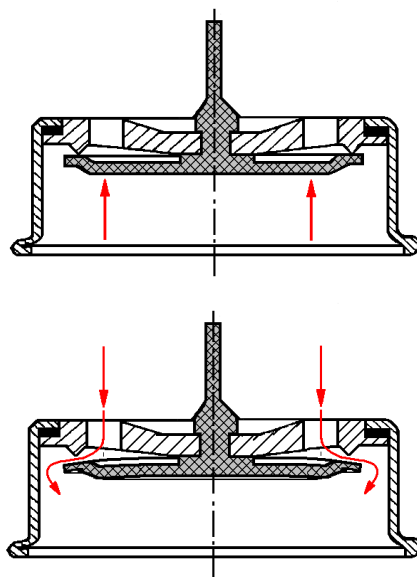
Rysunek nr 4.9. Zasada działania zaworu zwrotnego maski oddechowej
