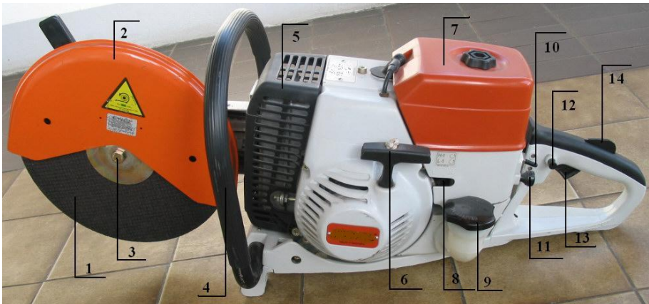
Fotografia nr 5.6. Budowa piły tarczowej
