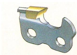
Rysunek nr 5.8. Zab tnący z węglików spiekanych (widia) stosowany w łańcuchach pił stosowanych przez użytkowników profesjonalnych podczas akcji ratunkowych, prac rozbiórkowych oraz cięcia drewna zanieczyszczonego.
