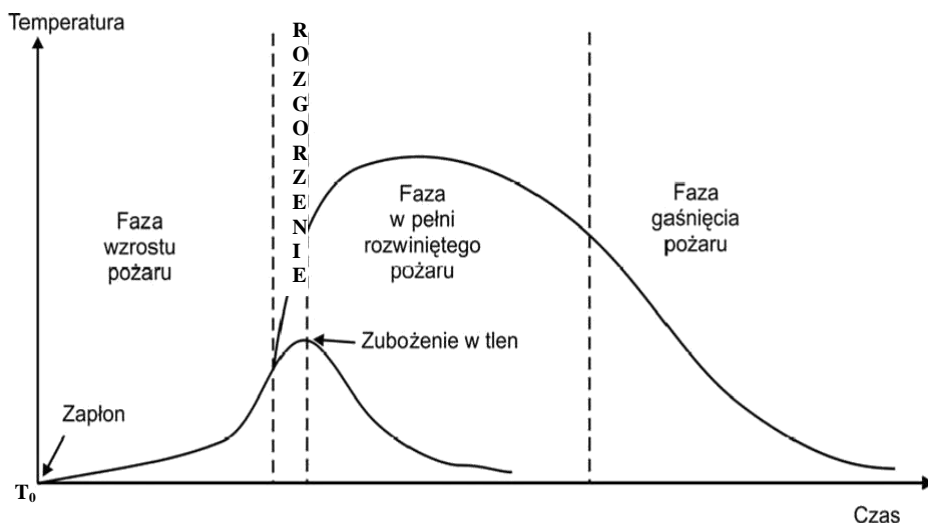
Rysunek nr 2.5. Hipotetyczny przebieg zmian temperatury pożaru w czasie trwania poszczególnych jego faz, dla warunków pożarowych niekontrolowanych działaniami gaśniczymi 22 ( T_0 – temperatura otoczenia)
