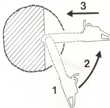
Rysunek nr 5.22. Rzaz wcinający
