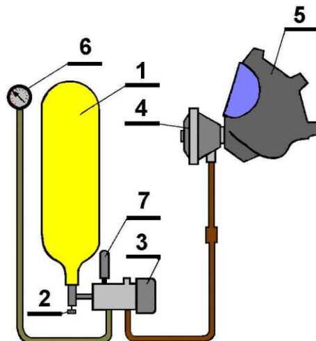
Rysunek nr 4.17. Aparat powietrzny z reduktorem o stopniach rozdzielonych
