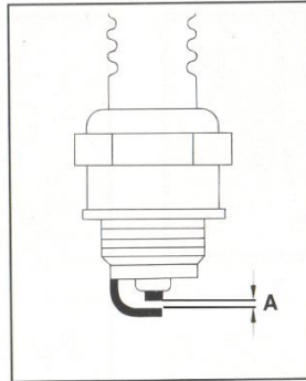
Rysunek nr 5.39. Pomiar odległości między elektrodami
